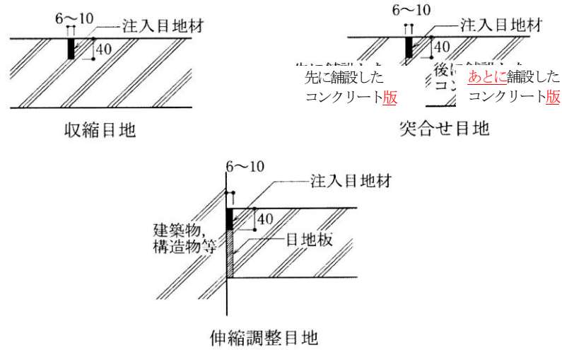
図22.5.1 目地の構造（単位：mm）
