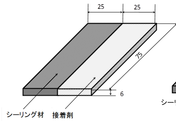
図 11.3.1 汚染性試験体
