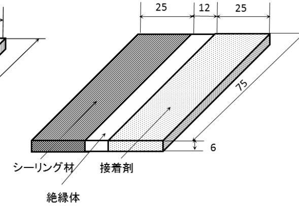
図 11.3.2 比較検討用試験体
