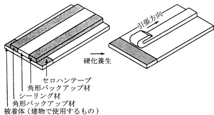
図9.6.1 簡易接着性試験
