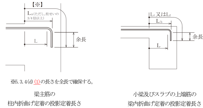
図 5.3.3 折曲げ定着の方法
