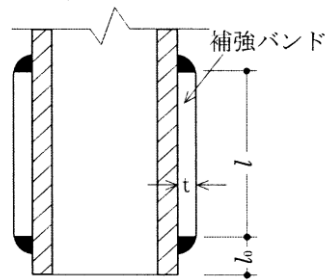
図 4.4.1 先端部補強
