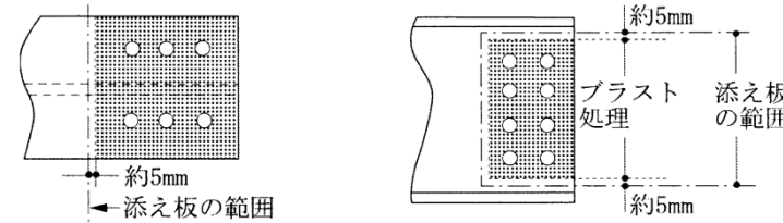
図 7.12.1 ブラスト処理の範囲
