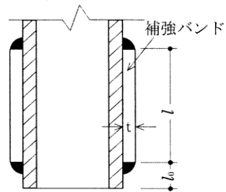
図 4.4.1 先端部補強
